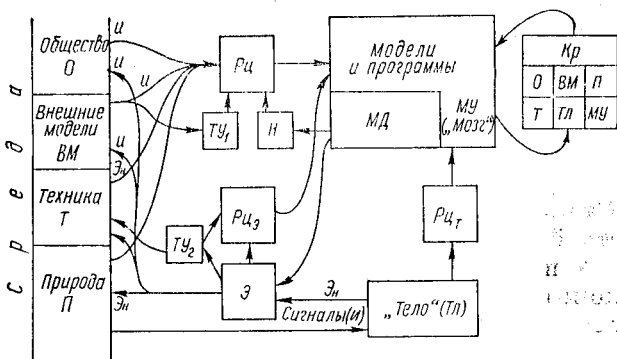
Рис. 21. Расширенная схема интеллекта.
