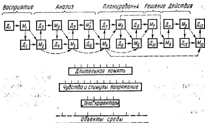
Рис. 29. Алгоритм функционального акта.
