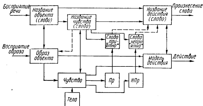
Рис. 36. Взаимоотношение моделей образов и моделей речи. Моделям образов объекта, чувств и действий соответствуют модели словесных эквивалентов. Между ними имеются прямые и обратные связи, так что они могут взаимно активировать друг друга.
